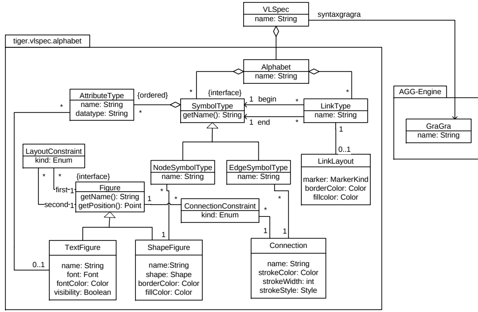
Fig. 4. Package tiger.vlspec
